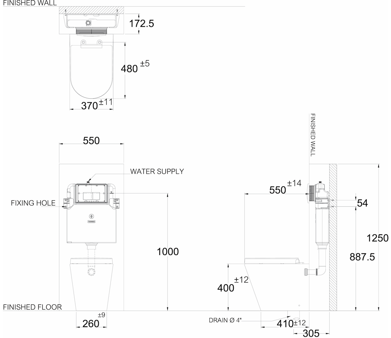
Dimension : โถสุขภัณฑ์ เมื่อประกอบกับชุดหม้อน้ำ Wall Faced ช้อนผนัง พร้อมปุ่มกดน้ำ รุ่น SP78
