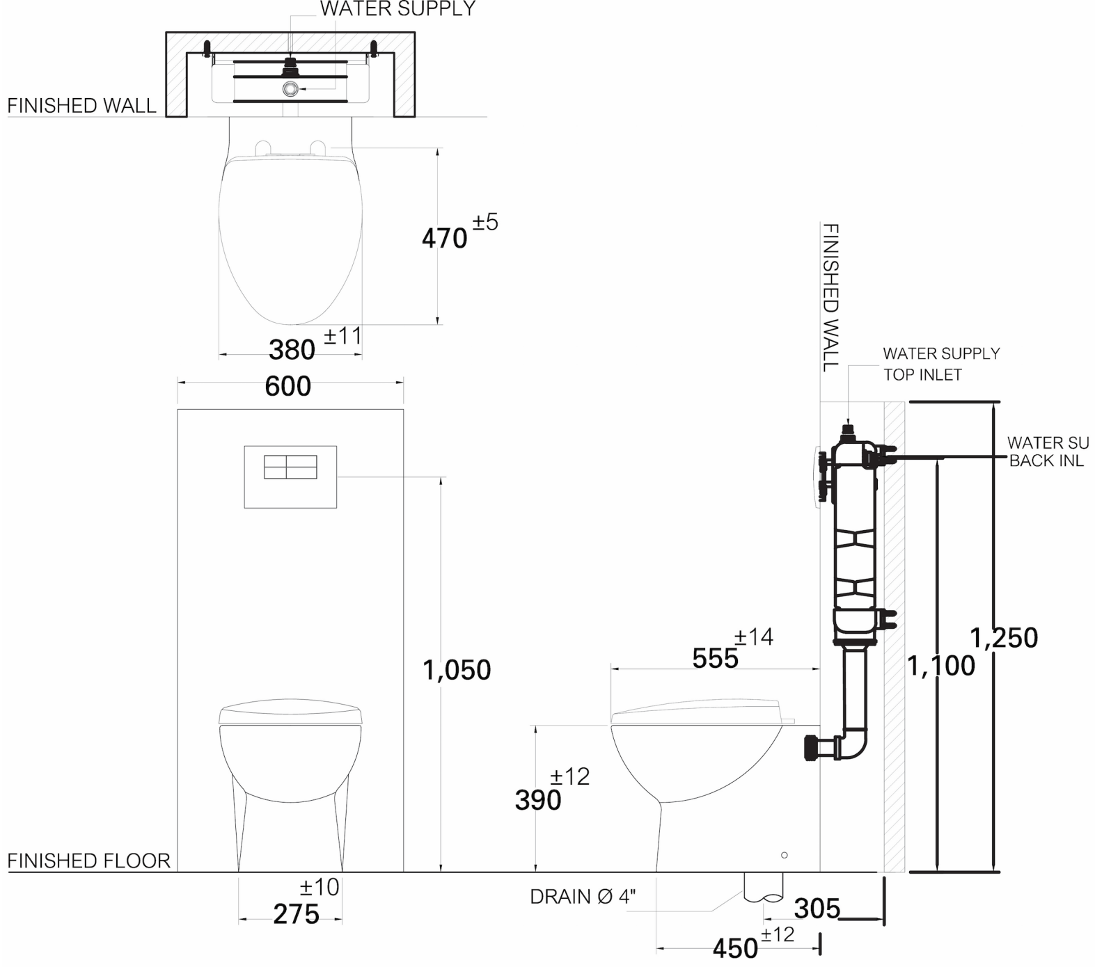
Dimension : โถสุขภัณฑ์ เมื่อประกอบกับชุดหม้อน้ำ Wall Faced ช้อนผนัง พร้อมปุ่มกดน้ำ รุ่น SP78
